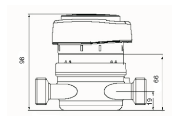
Widok z boku - wersja rozłączna (PolluCom E/S) Całkowita wysokość PolluCom E/SL wynosi 120mm
